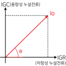
누설전류 분석 벡터 해석도
